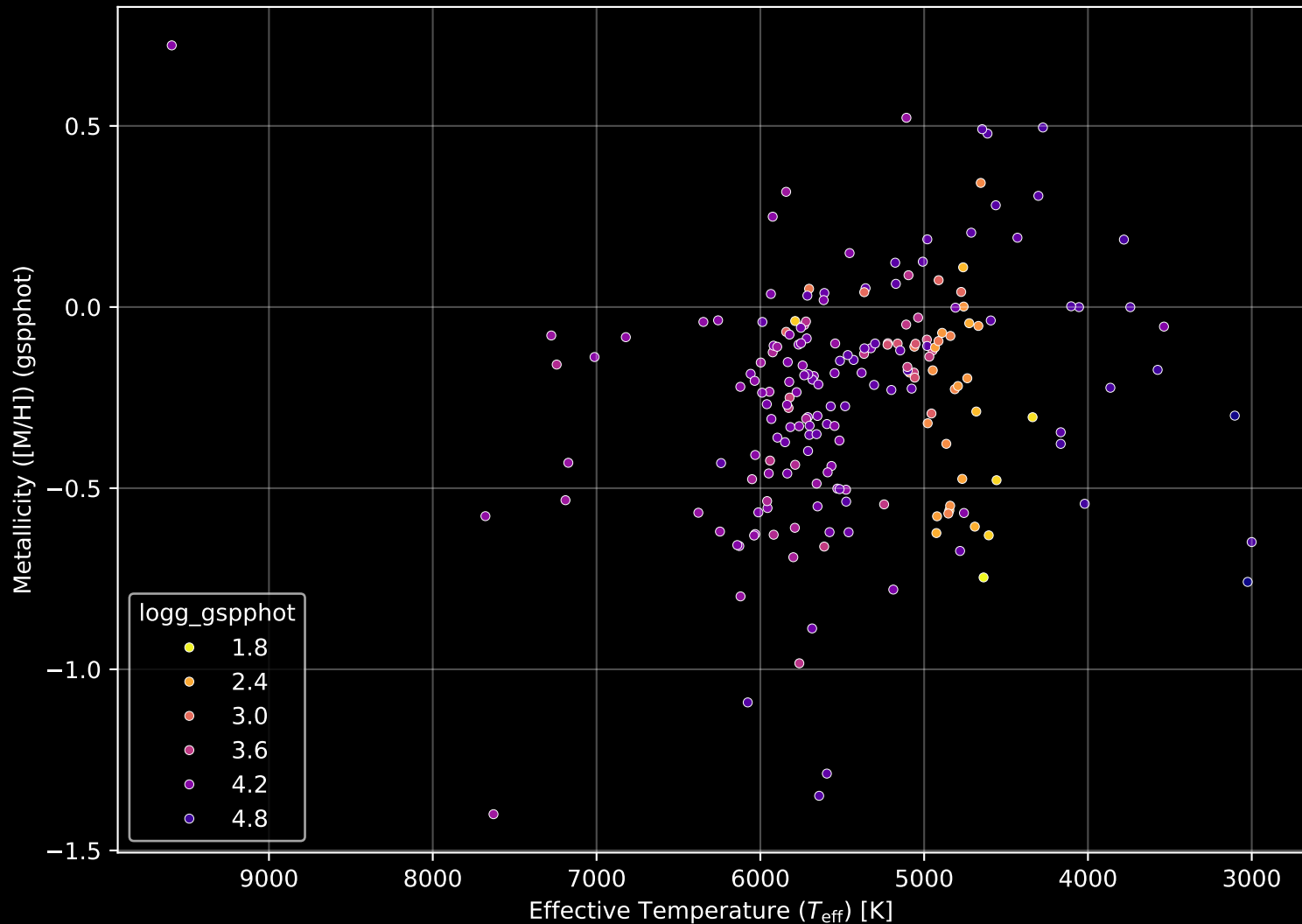
APOGEE DR17 Field: [196+35_MGA] Stellar Population Parameters (n= 198)
